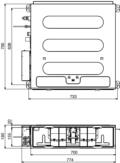
Ед. изм.: мм
